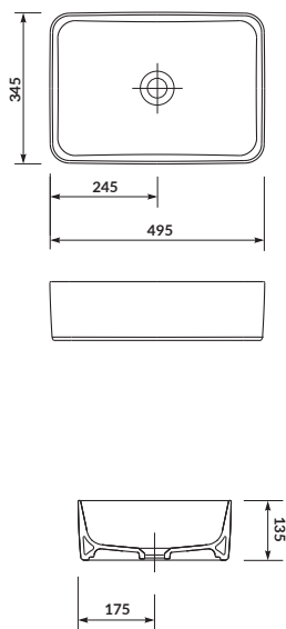
K114-001 UMYWALKA NABLATOWA CREA 50 CREA 50 COUNTERTOP WASHBASIN RECTANGULAR
