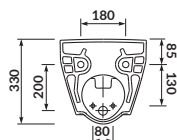
S701-357 SET B144 PISUAR CREA CLEANON SET B144 CREA CLEANON URINAL
