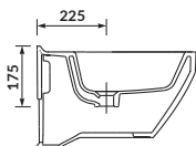
S701-357 SET B144 PISUAR CREA CLEANON SET B144 CREA CLEANON URINAL
