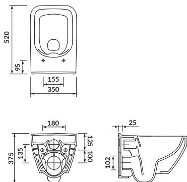
K114-016 MISKA ZAWIESZANA CREA CLEANON PROSTOKĄTNA CREA WALL HUNG BOWL CLEANON RECTANGULAR
