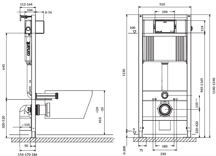
S97-050 STELAŻ PODTYNKOWY AQUA 72 PNEU S QF CONCEALED CISTERN FRAME AQUA 72 PNEU S QF
