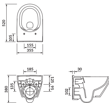
K114-015 MISKA ZAWIESZANA CREA CLEANON OWALNA CREA WALL HUNG BOWL CLEANON OVAL
